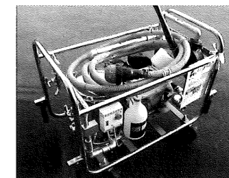
特注製作の緊急用浄水装置。年に一度、作動させて職員に使い方を教えている
